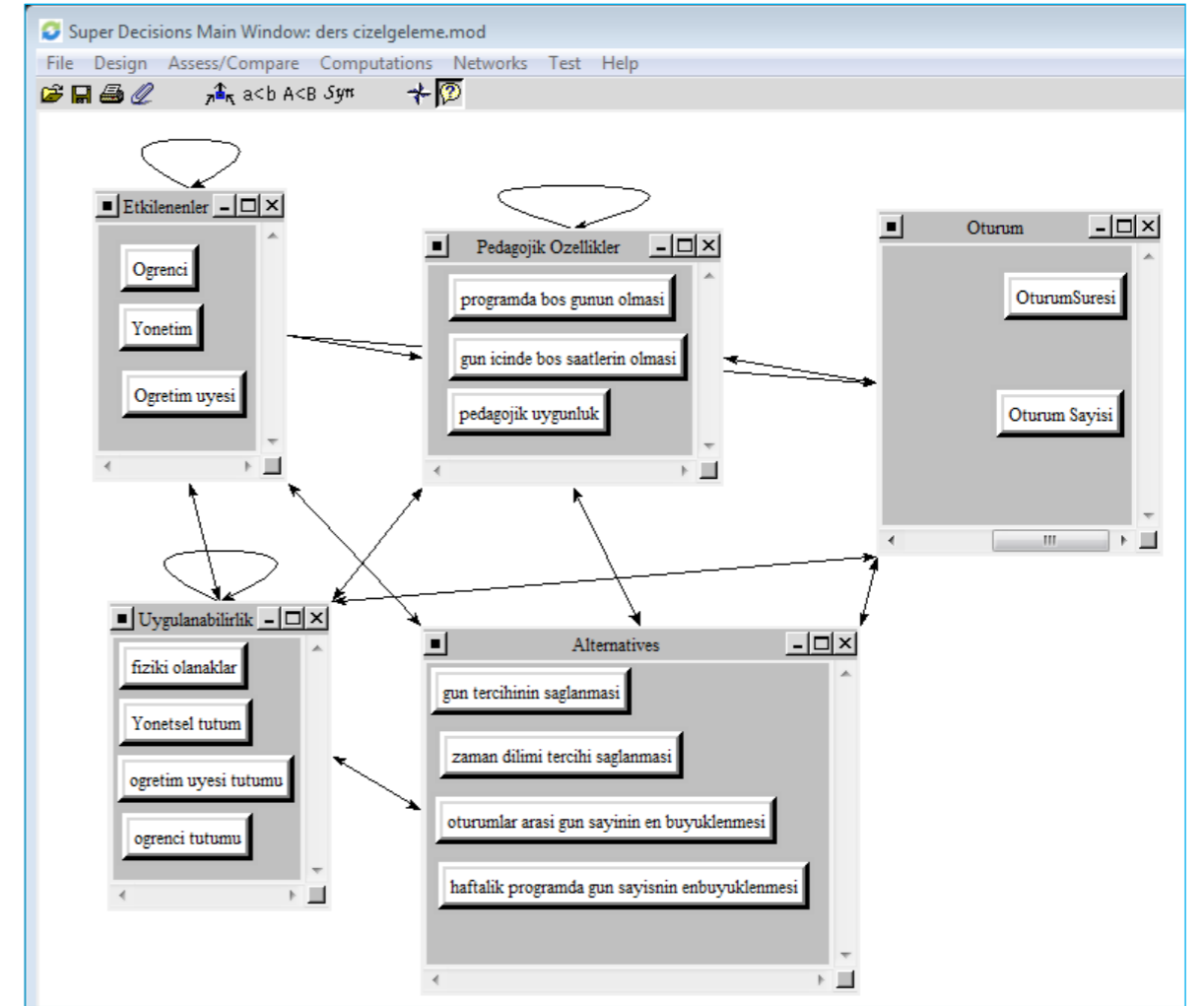
Şekil 1. Ders Çizelgeleme Problemi İçin Geliştirilen ASS Modeli
